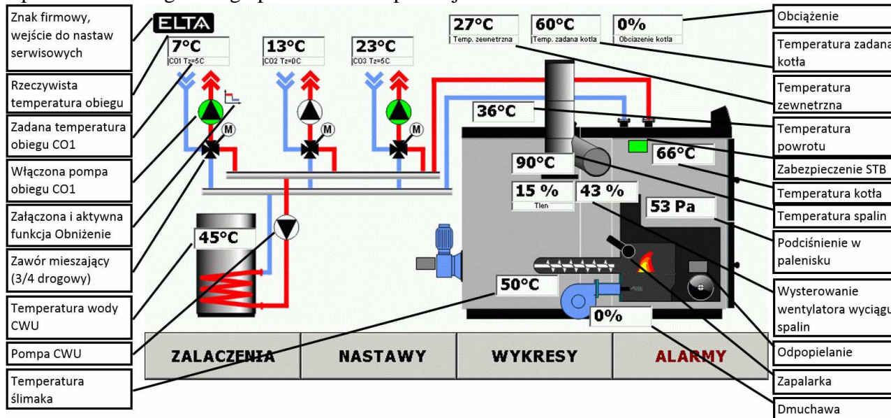
Rys. 15.1 Opis ekranu głównego.
