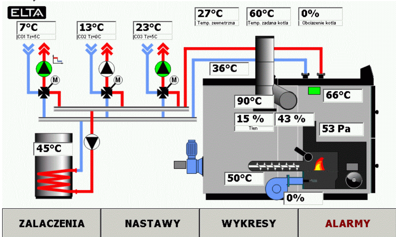
Rys. 3.1 Ekran główny DLC-200S.
